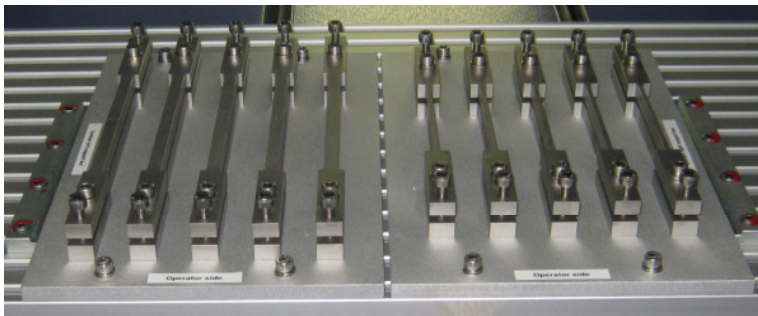
Universalspannzeuge 201-125 und 201-124 für 5 Normstäbe
